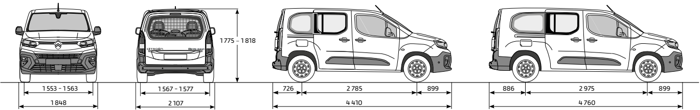
Wszystkie wymiary w mm
